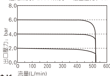
低壓型溢流特性
