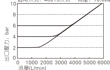
高壓型溢流特性
