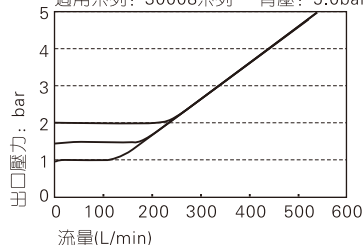
中壓型溢流特性
