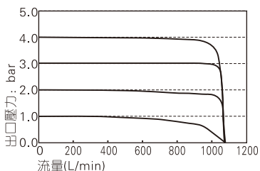
高壓型流量特性
