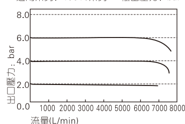
低壓型溢流特性
