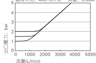
中壓型溢流特性
