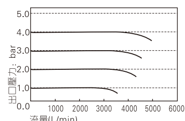
高壓型流量特性
