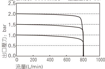
中壓型流量特性
