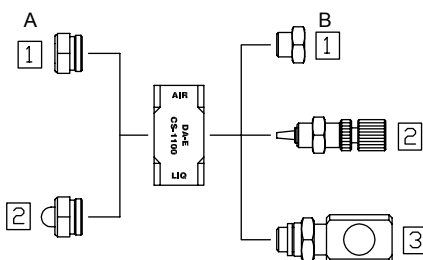
組合圖
