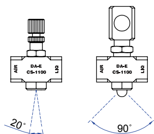
噴頭角度
