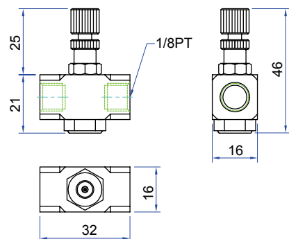
外觀尺寸
